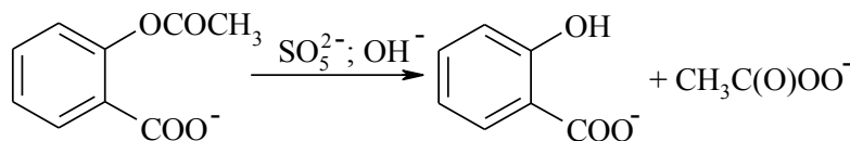
Рис. 8. Хімізм пергідролізу ацетилсаліцилової кислоти
