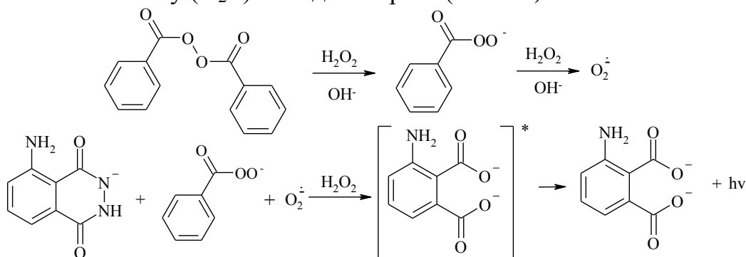
Рис. 11. Хімізм пергідролізу бензоїлу пероксиду та окиснення люміналу
