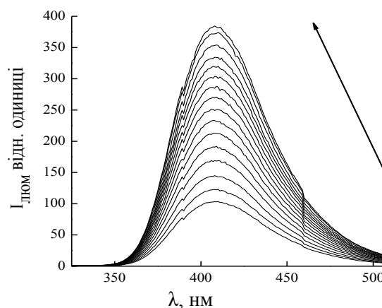
Рис. 10. Спектри флуоресценції продукту пергідролізу D,L\text{-лізину ацетилсаліцилату} в присутності KHSO_5 . c(D,L\text{-лізину ацетил-саліцилату})=28,8 мкг/мл; c(KHSO_5)=3,6 \cdot 10^{-3} моль/л; рН=10,5.
