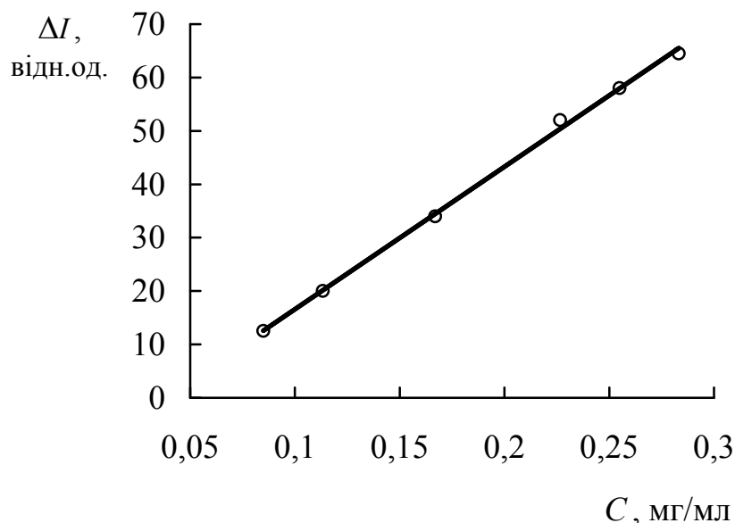
Рис.3. Градуювальна залежність кількісного визначення A за ефектом інгібування XЛ в системі H_2L - H_2O_2 - (A) - Het
