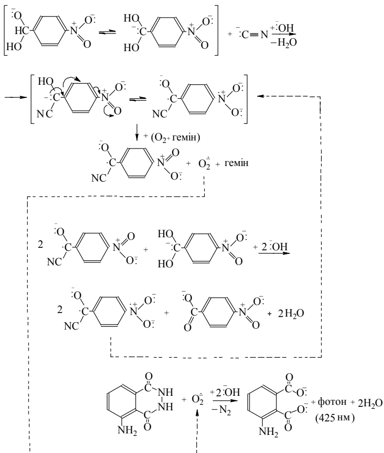
Рис. 3. Послідовність реакцій у автокаталітичній системі n -НБА–СН–О 2 –гемін–люмінол.
