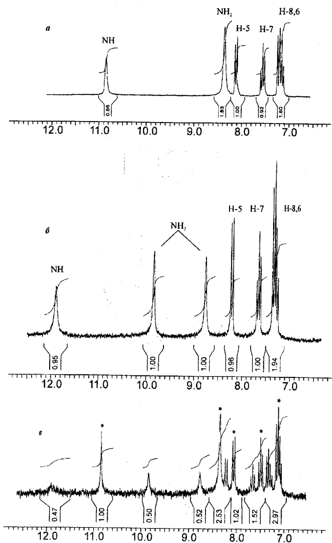
Рис. 1. Фрагменты спектров ПМР: эфира 4 (а); кислоты 12 (б) и их смеси в соотношении 2:1 (в), где звездочками отмечены сигналы протонов эфира 4.
