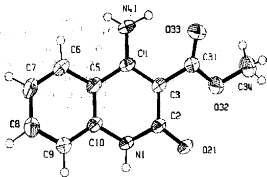
Рис. 2. Эллипсоиды тепловых колебаний и нумерация атомов эфира 2.
