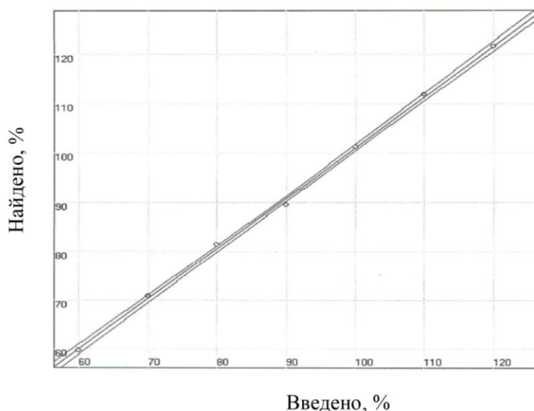
Рис. 1. График зависимости площади пиков от концентрации фенобарбитала в нормализованных координатах
