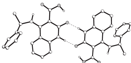
Рис. 3. Центросимметричные димеры, образованные за счет межмолекулярных водородных связей N(1)-H(1N)\dots O(1)' ( 1 - x, 1 - y, -z ) в кристалле рацемата.
