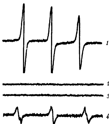
Рис. 4. Спектры ЭПР липофильного зонда (2): 1 – в водном растворе; 2 – смеси зонда и уширителя; 3 – смеси зонда, уширителя и УНТ; 4 – зонда в суспензии УНТ
