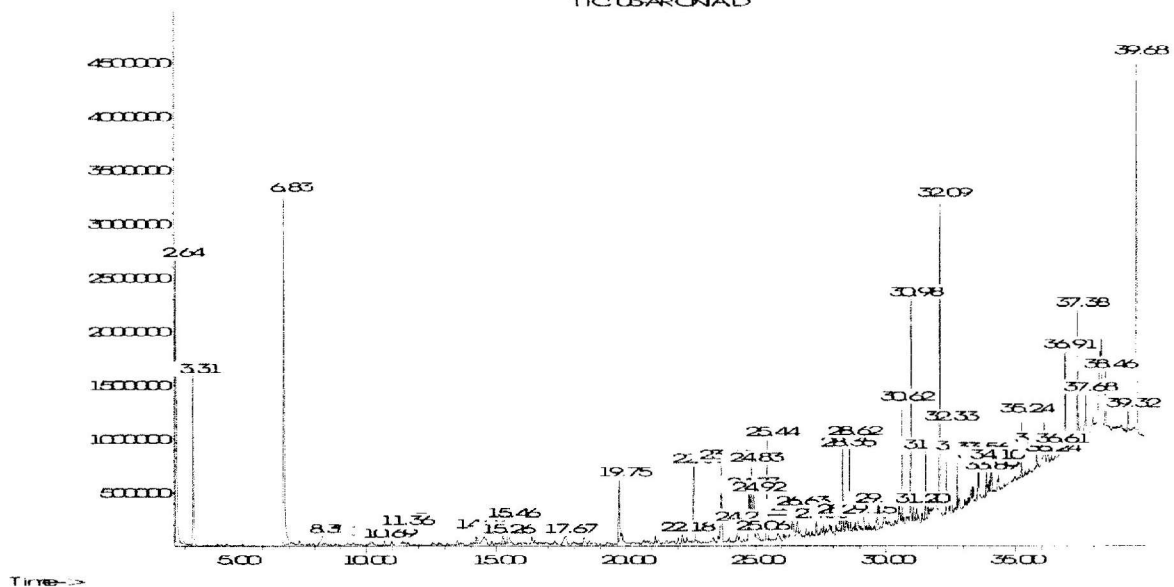
Рис. 1. Хроматограма летких речовин листя аронії чорноплідної.
