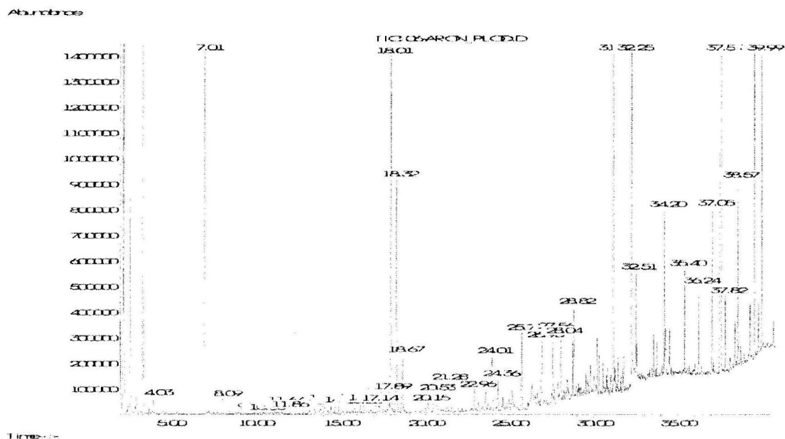
Рис. 2. Хроматограма летких речовин плодів аронії чорноплідної.
