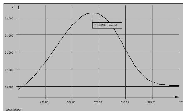
Рис. 1. Спектр поглинання аналітичного розчину.
