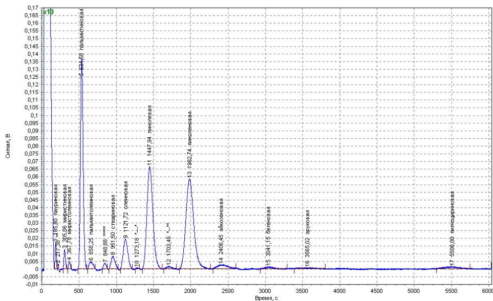
Рис. 1. Хроматограмма жирнокислотного состава листьев мать-и-мачехи
