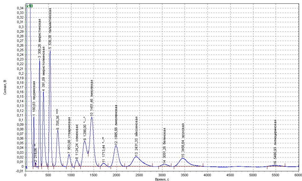
Рис. 2. Хроматограмма жирнокислотного состава цветков мать-и-мачехи
