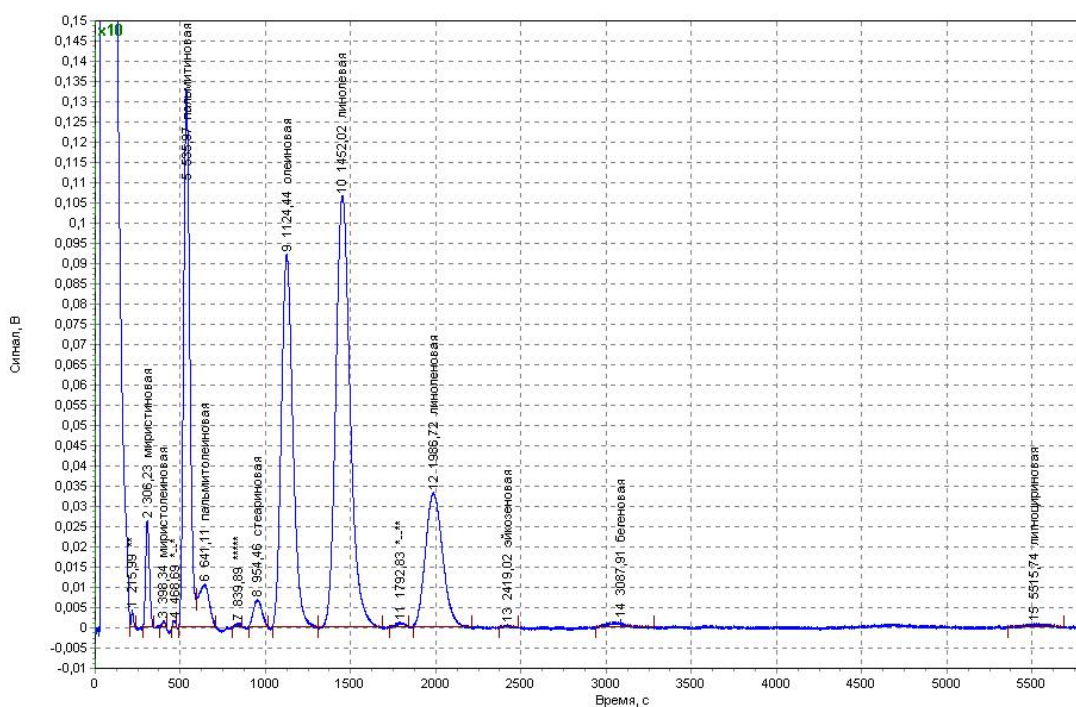
Рис. 3. Хроматограмма жирнокислотного состава корней мать-и-мачехи
