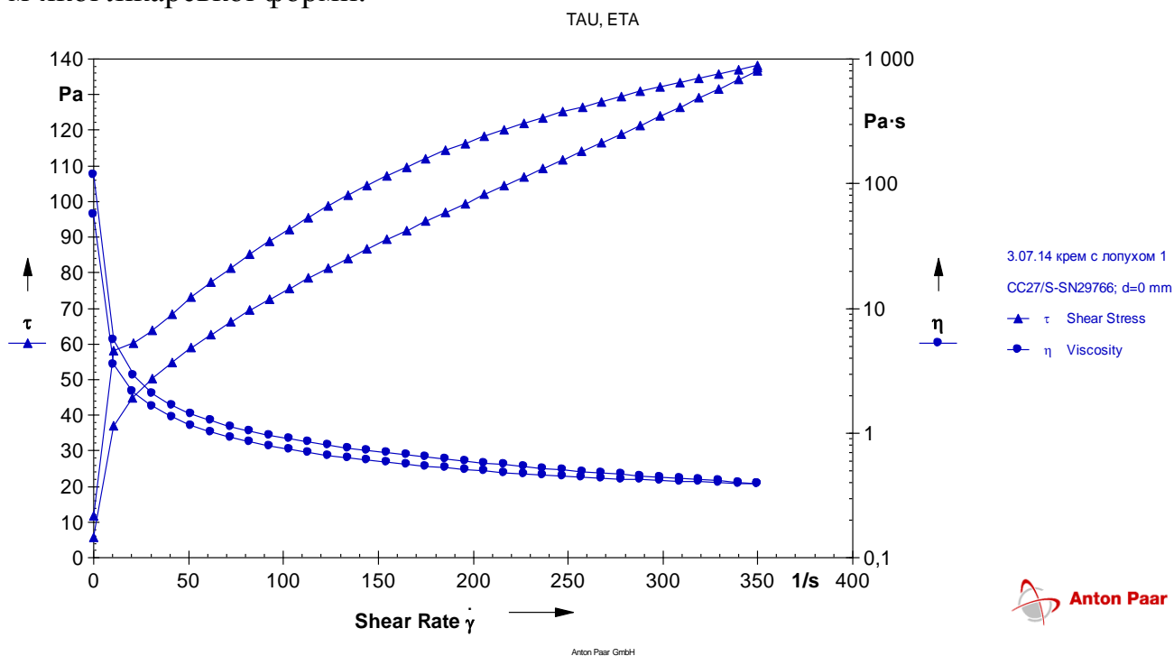
Рис. 1 Реограма плинину гелю та залежність структурної в'язкості гелю від швидкості зсуву
