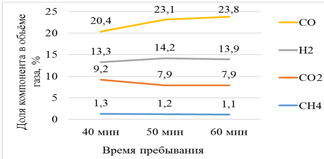
Рис 3. Изменение состава генераторного газа после газификации полукокса при изменении времени пребывания полукокса в зоне газификации.
