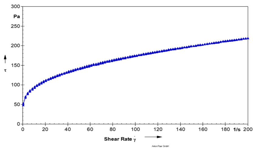
Рис. 3.18. Реограма зразка з 1 % вмістом Seriplus-400
