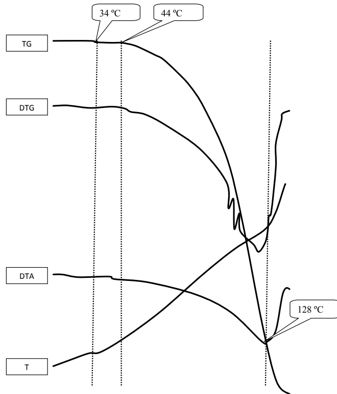
Рис. 3. Дериватограма глюкозаміну гідрохлориду
