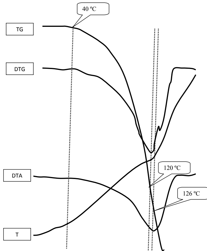
Рис. 4. Дериватограма лавандової олії
